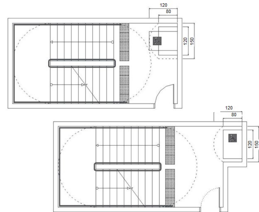
Figura 52 –Área de resgate junto a escadas e em espaço confinado
