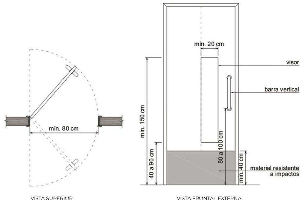
Figura 58 – Características das portas tipo vai-vem
