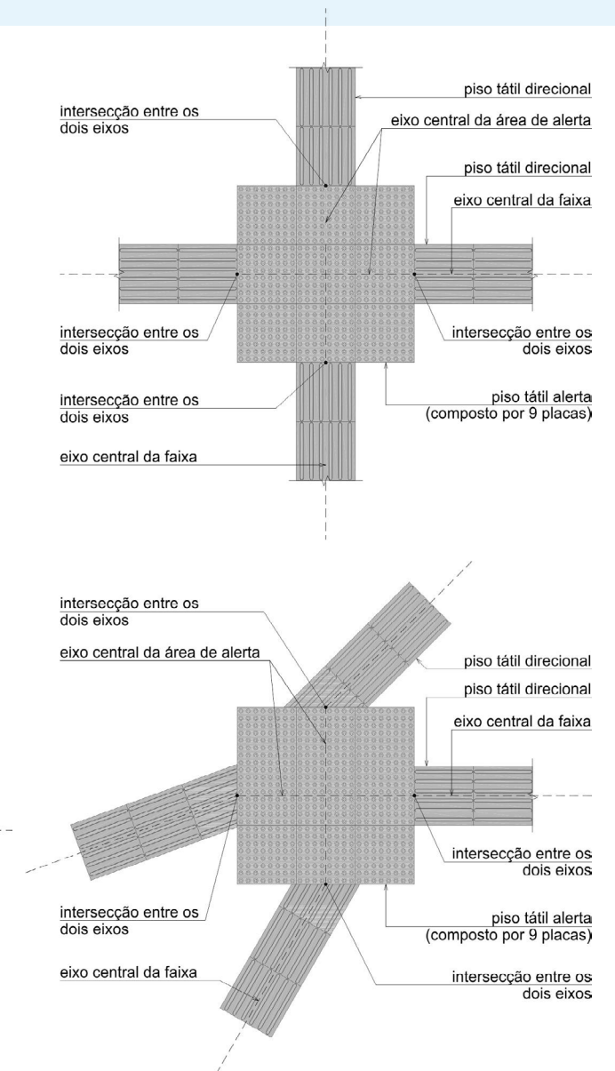
Figura 27 – Mudança de direção – encontro de quatro faixas
