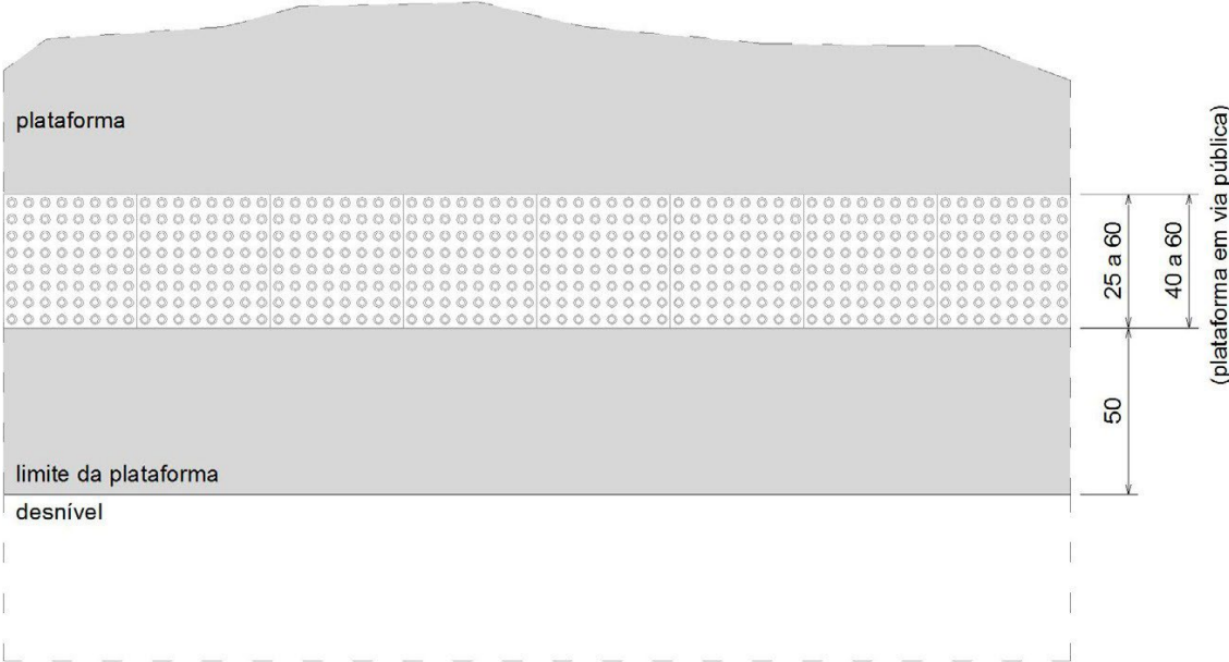
Figura 40 – Sinalização de limite de plataforma
