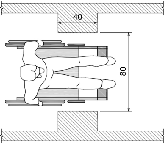
Figura 44 – Transposição de obstáculos isolados
