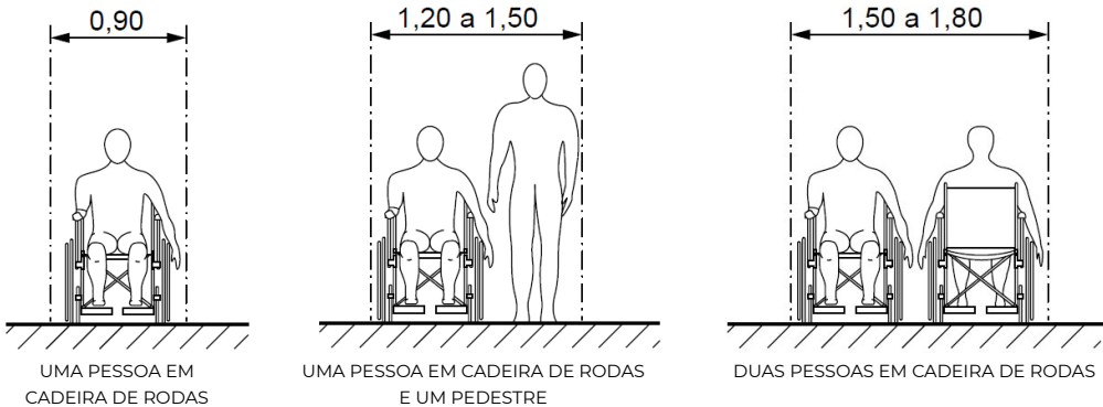
Figura 13 - Largura para deslocamento em linha reta
