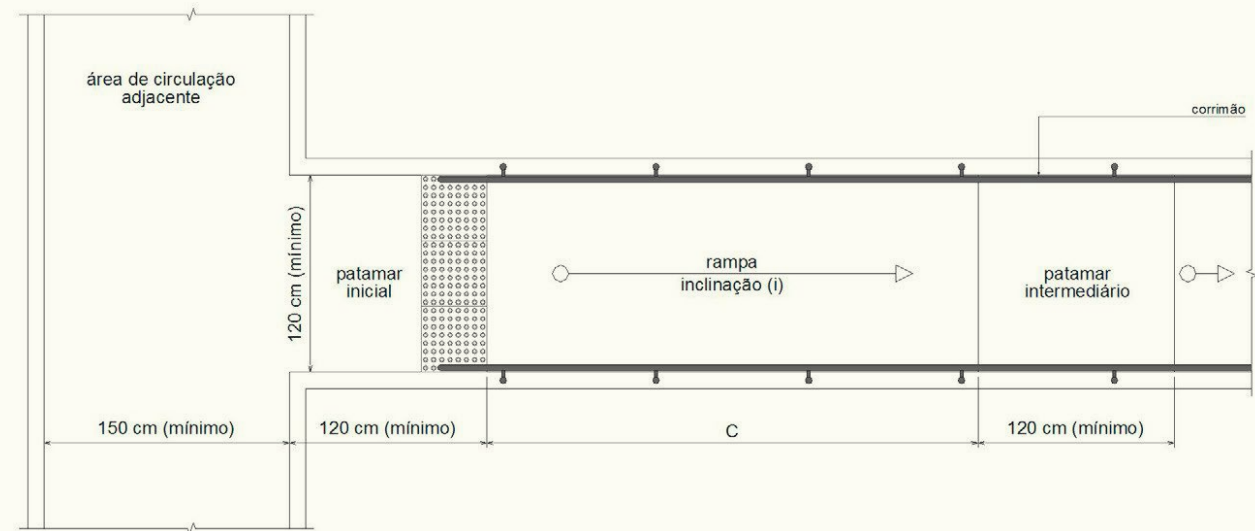
Figura 50 – Patamar de rampa - exemplo
