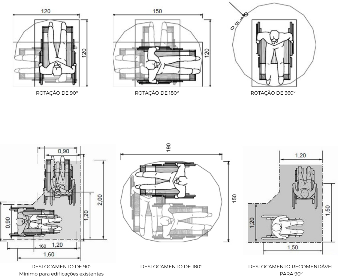
Figura 12 - Área de manobra com deslocamento
