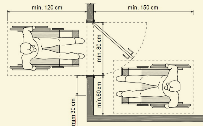
Figura 55 – Distâncias mínimas para abertura de portas
