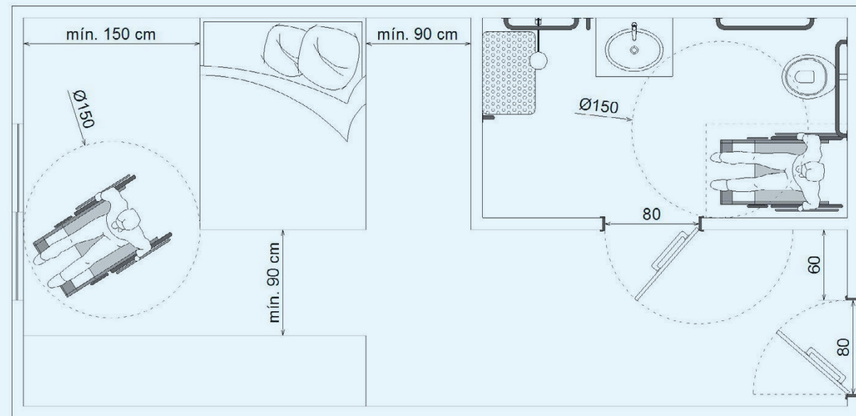
Figura 73 – Dormitório – Vista Superior
