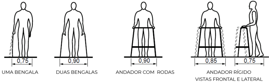
Figura 7 – Dimensões referenciais para deslocamento de pessoas com bengala e andador
