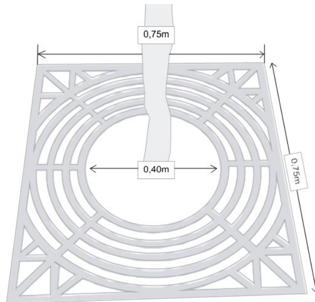
Figura 42 - Protetor de base
