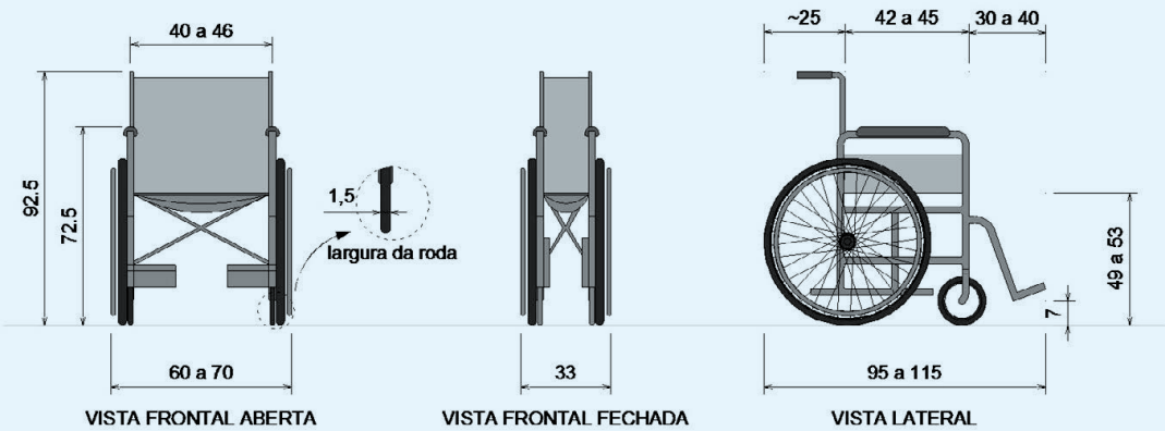
Figura 6 - Cadeira de Rodas (dimensões em centímetros)
