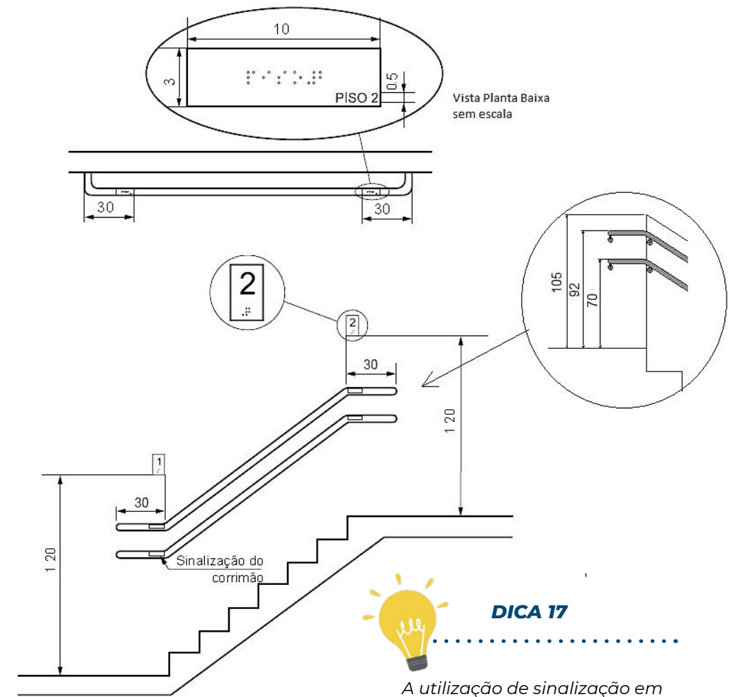
Figura 69 – Instalação de guarda-corpo e corrimão
