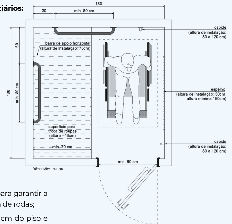
Figura 68 – Vestiário – Vista superior
