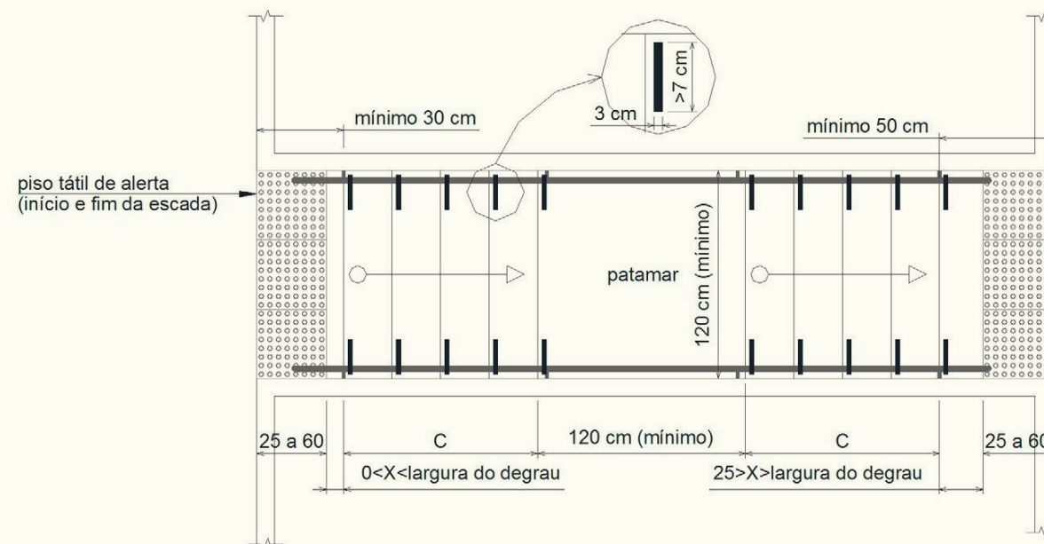
Figura 51 – Detalhes construtivos de escada (L < 240 cm)
