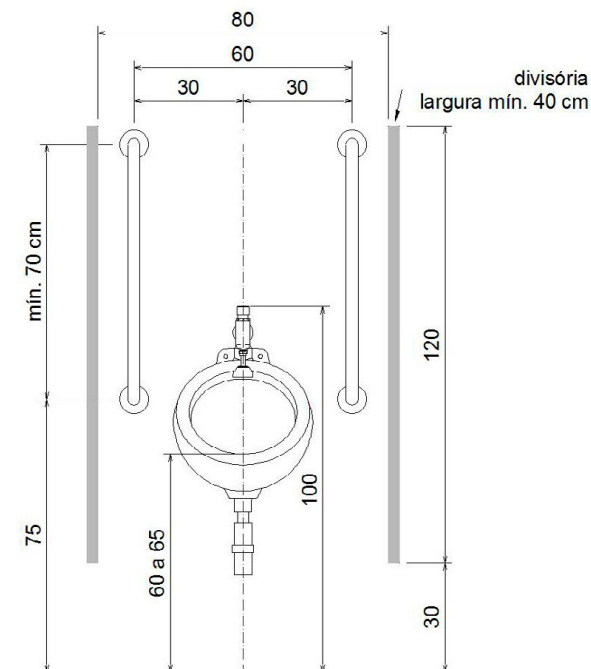
Figura 63 – Vista Frontal - Mictórios
