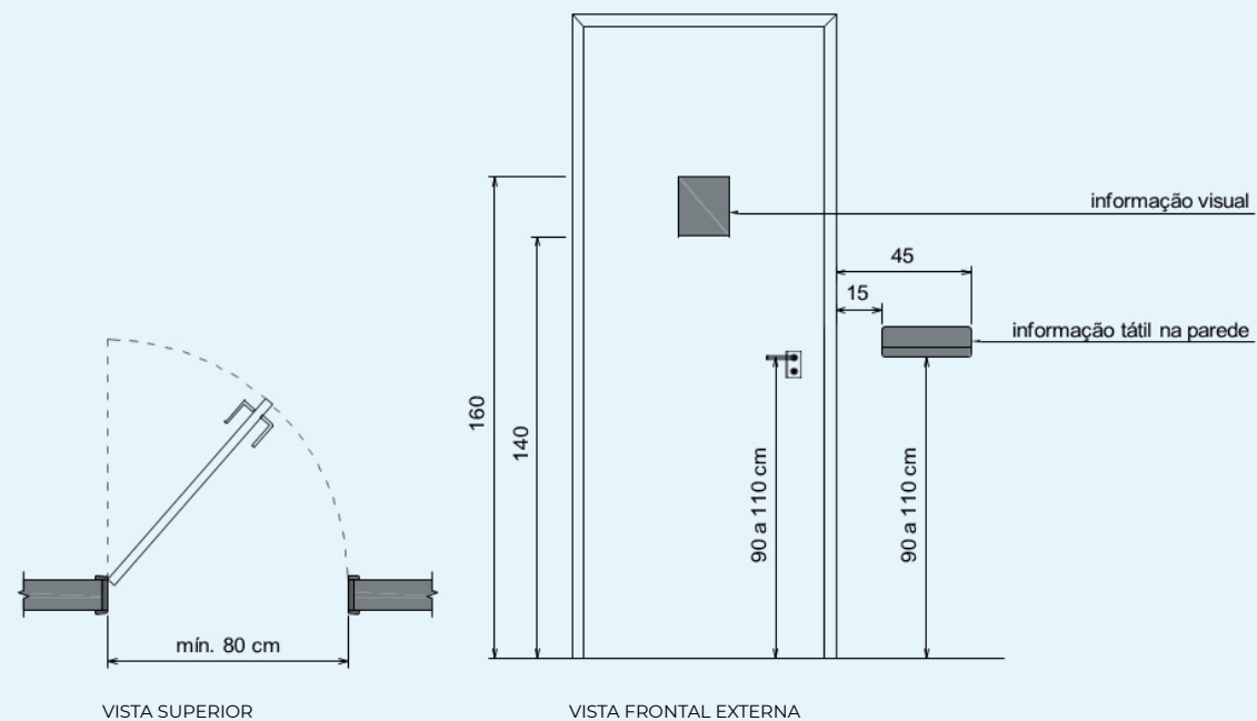
Figura 56 – Características das portas
