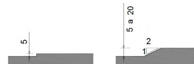
Figura 46 – Tratamento de desníveis até 20 mm
