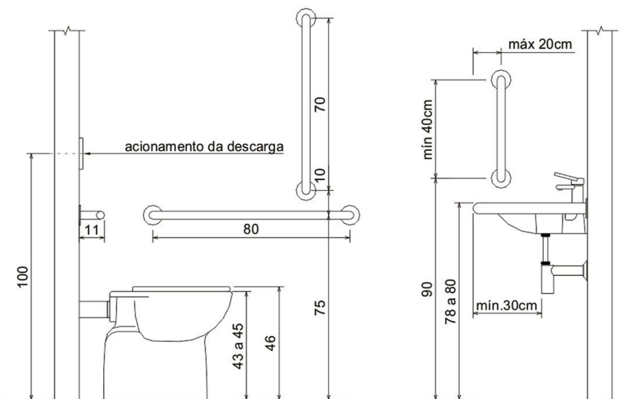
Figura 62 – Vista lateral do sanitário acessível
