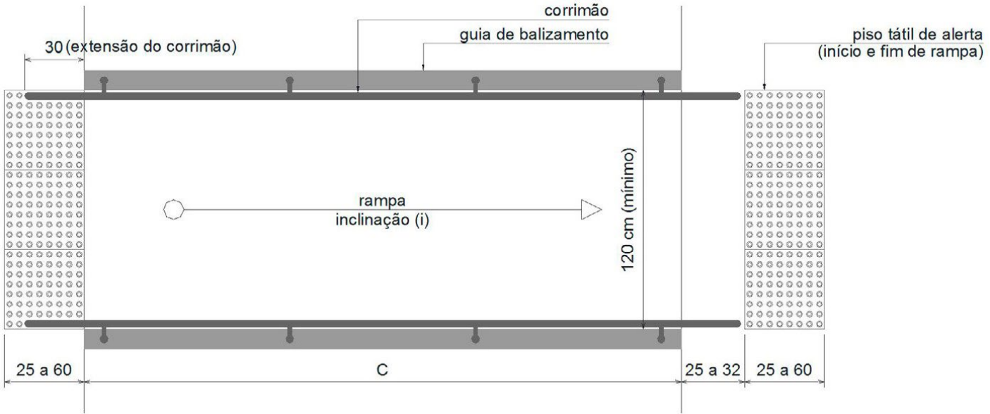
Figura 48 – Detalhes construtivos da rampa – vista superior
