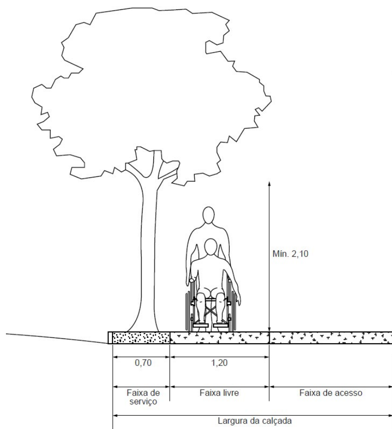
Figura 15 – Faixas de uso da calçada.
