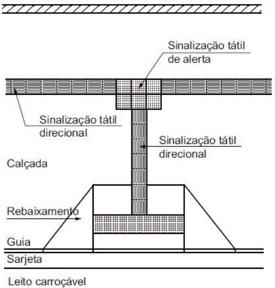
Figura 29 – Travessia de pedestres
