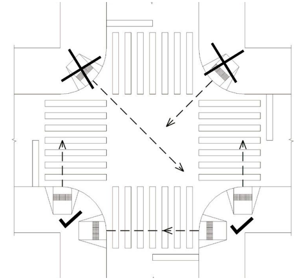
Figura 28 – Recomendação para instalação da travessia de pedestres em esquinas
