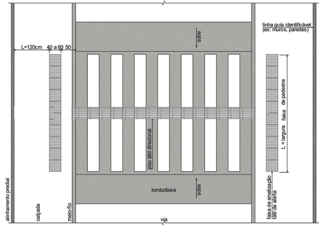
Figura 32 – Travessia com lombafaixa
