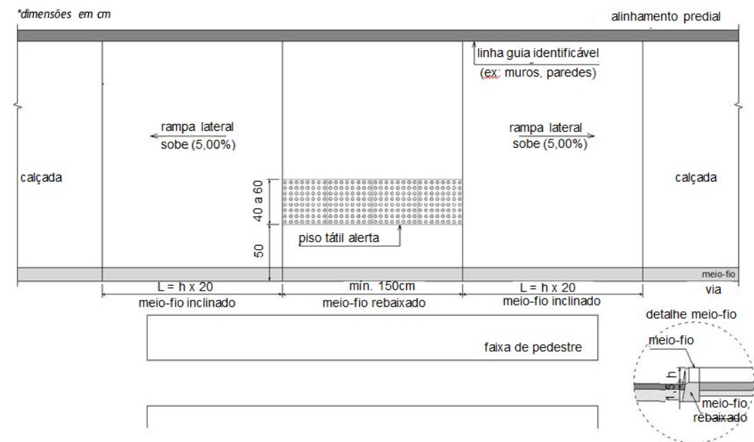
Figura 31 – Travessia de pedestres para largura remanescente \leq 120 cm e inclinação de piso < 5\%
