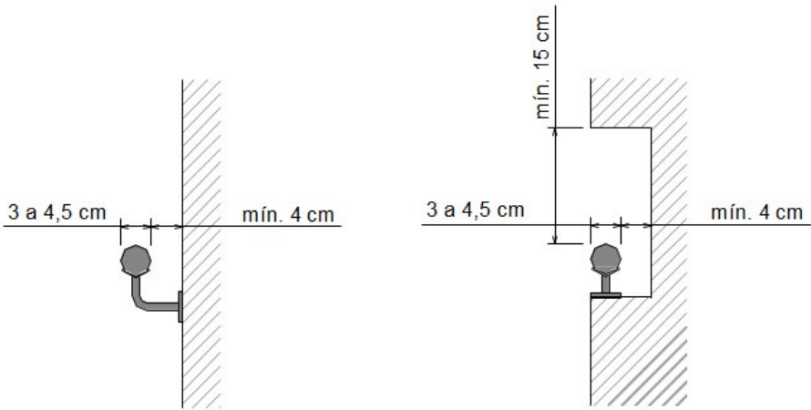
Figura 70 – Detalhes do corrimão
