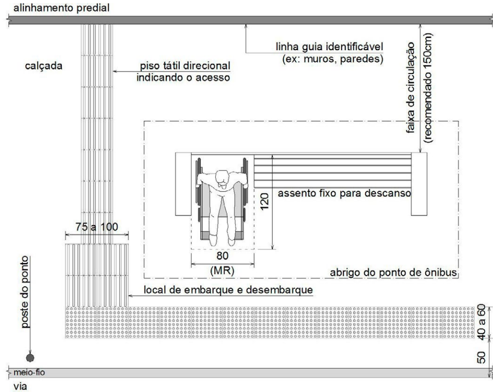
Figura 41 – Local de embarque de transporte público
