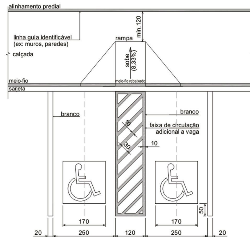
Figura 38 – Vaga de estacionamento em 90° com a calçada
