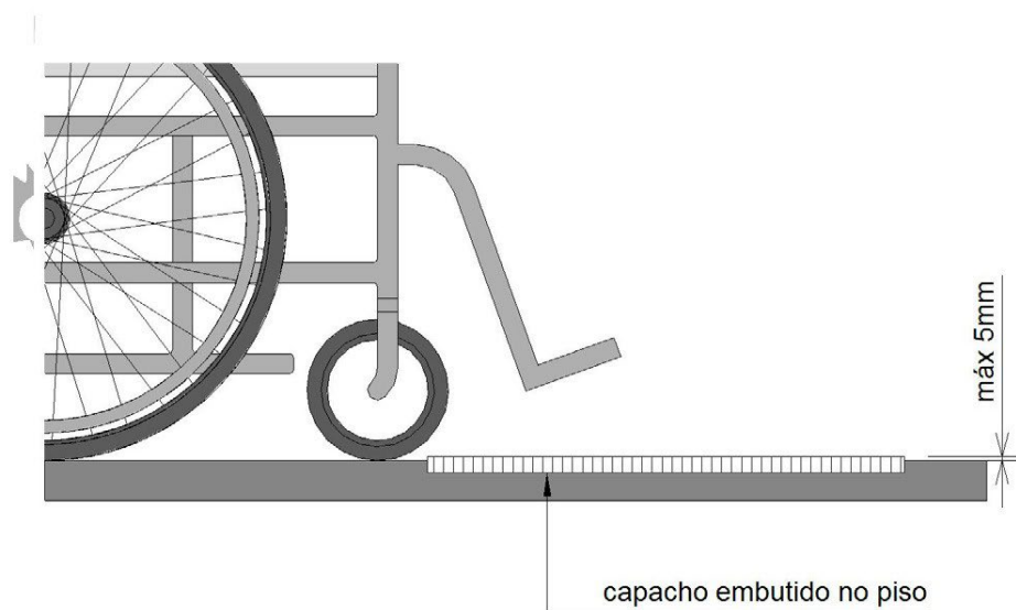
Figura 45 – Instalação de capachos embutidos
