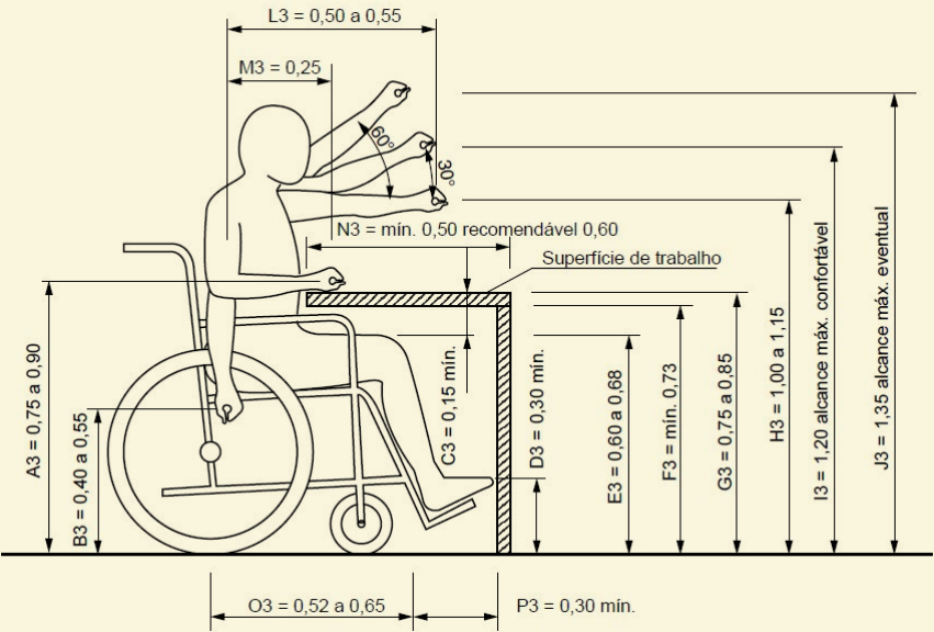
Figura 14a - Alcance manual de usuários de cadeira de rodas.
