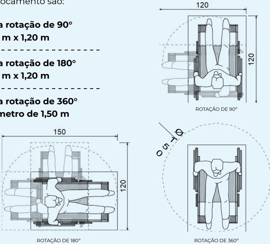
Figura 11 - Área de manobra sem deslocamento
