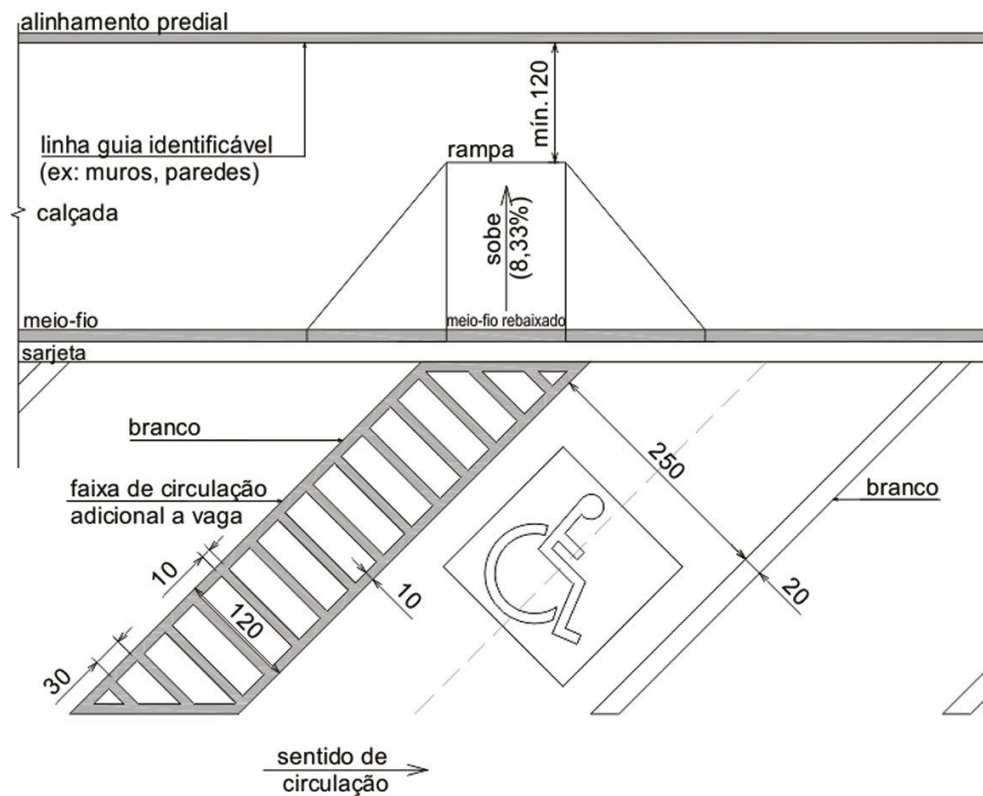
Figura 37 – Vaga de estacionamento a 45° com a calçada
