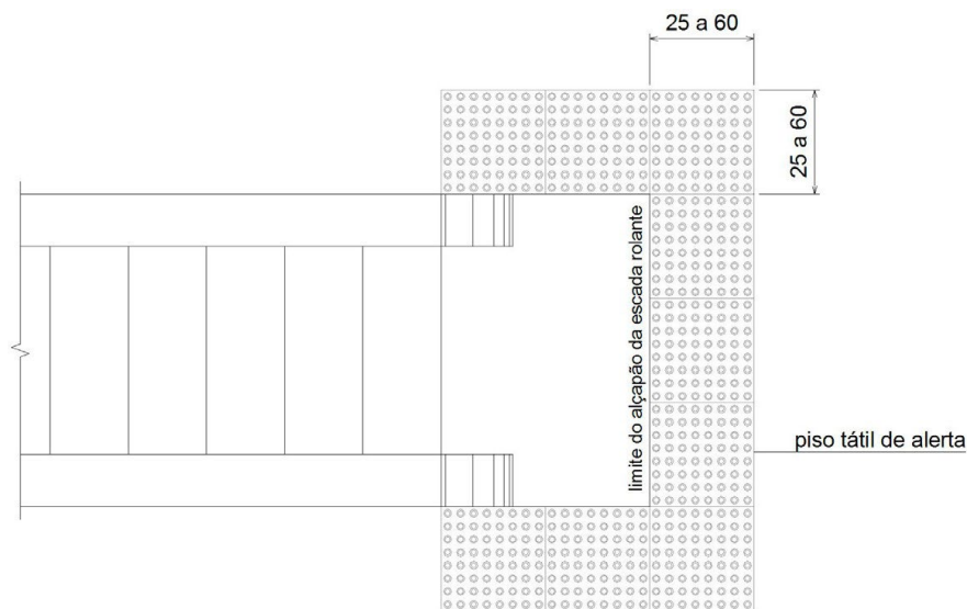
Figura 54 – Sinalização para escada rolante
