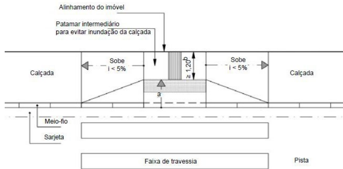
Figura 30 – Rebaixamento de calçadas estreitas.
