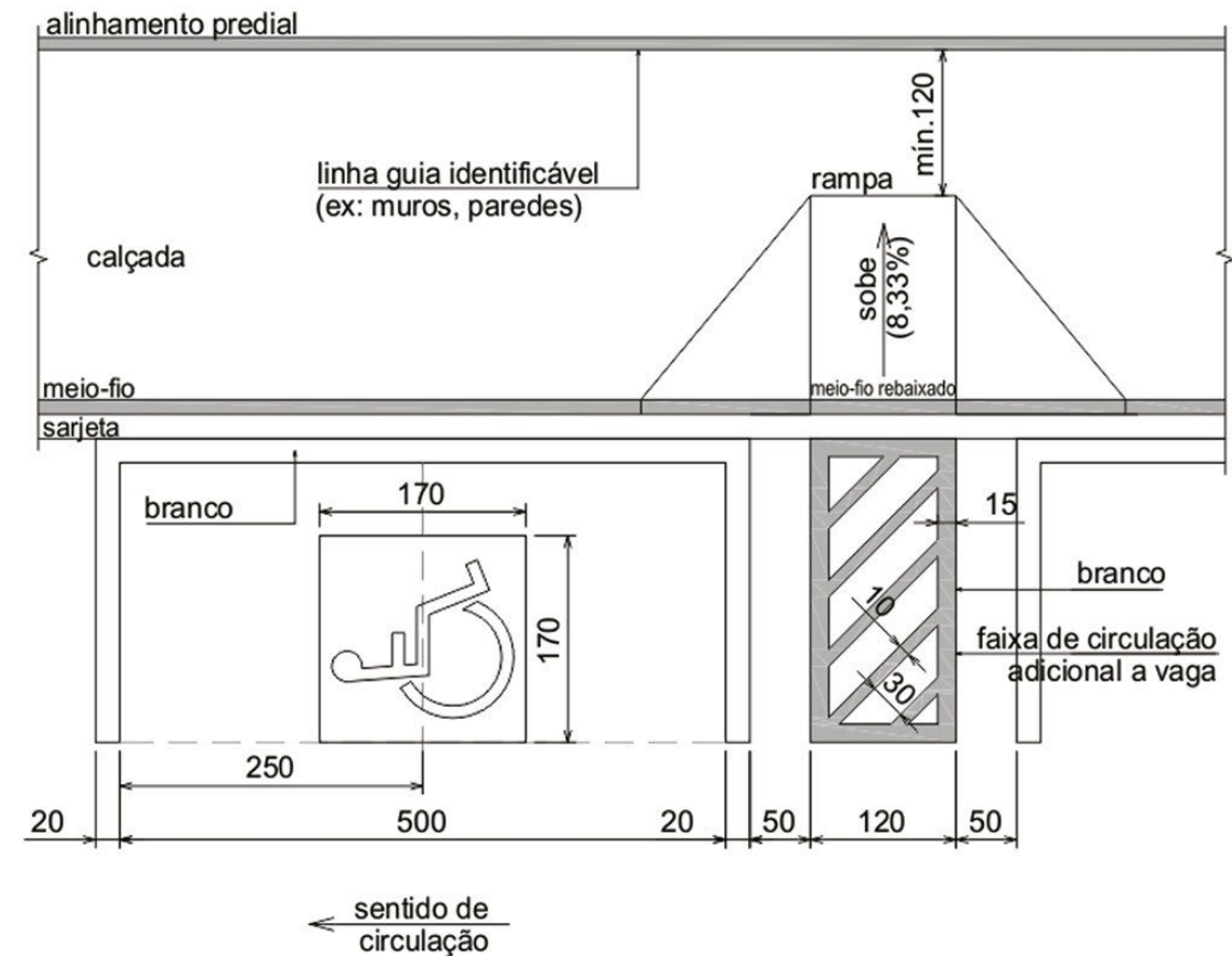
Figura 36 – Vaga de estacionamento paralela a calçada
