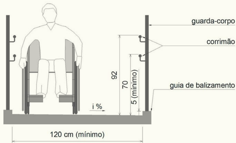
Figura 49 – Detalhes construtivos da rampa – vista frontal
